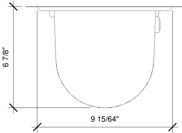
1 PH235 TOP 3" = 1'-0"
